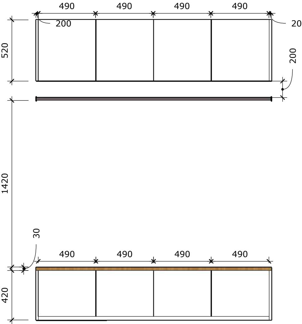
Čelný pohľad
