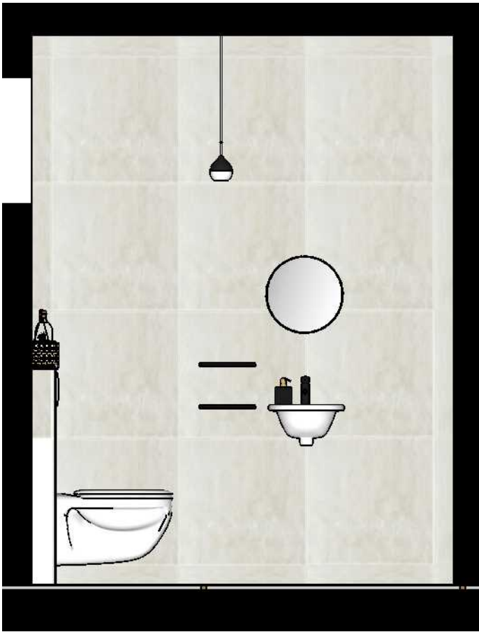
REZOPOHĽAD D
