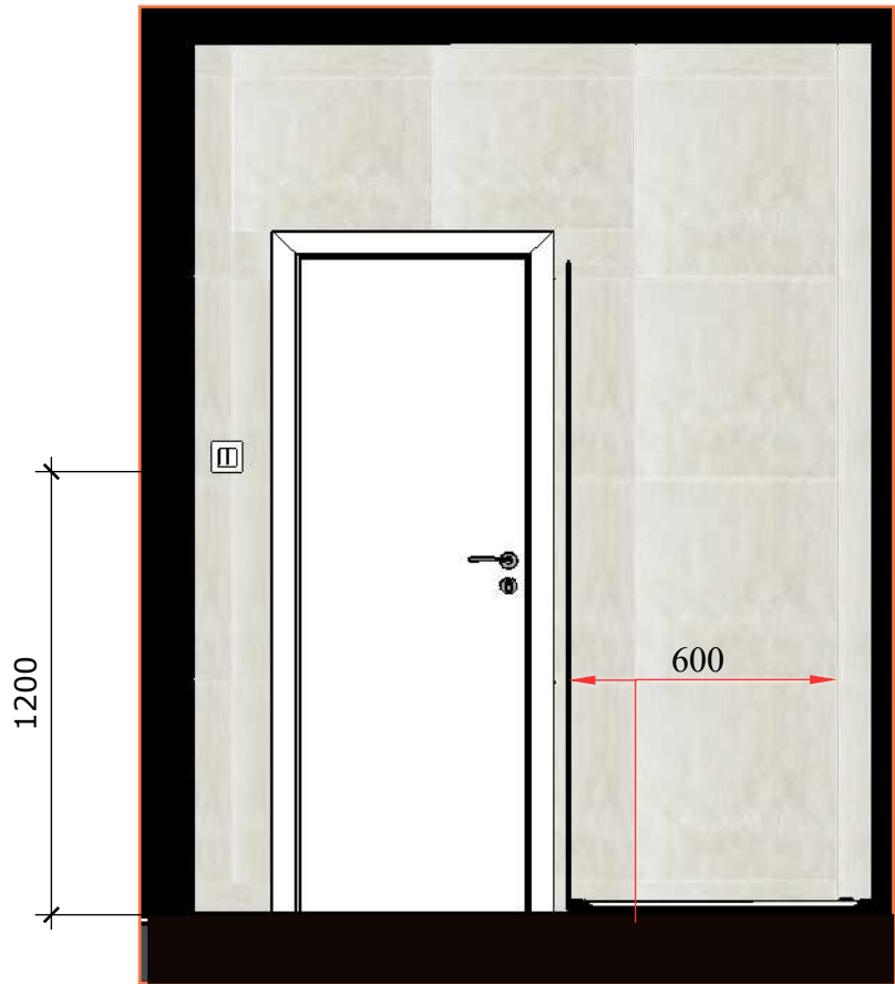
REZOPOHLAD D
