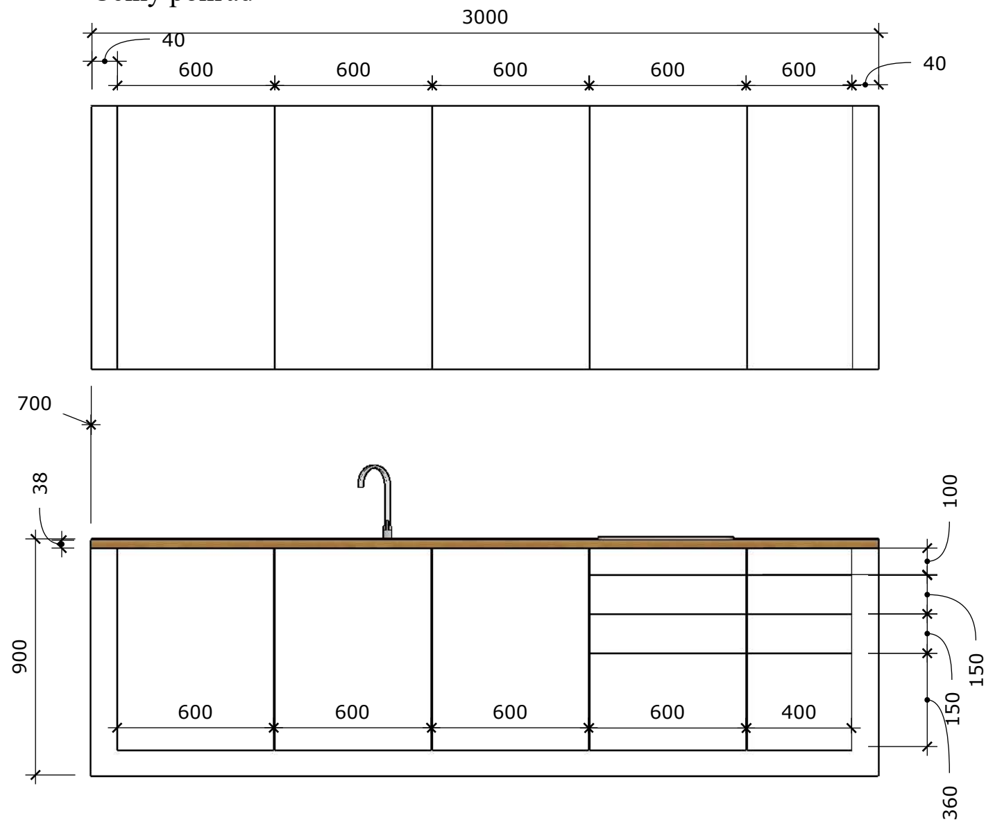
Čelný pohľad
