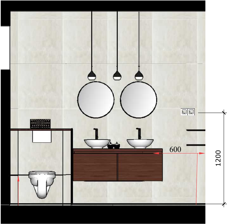
REZOPOHĽAD A
